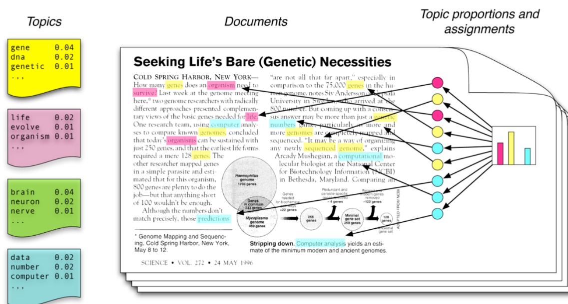
Figura 5 – Atribuição de tópicos a um documento em LDA
