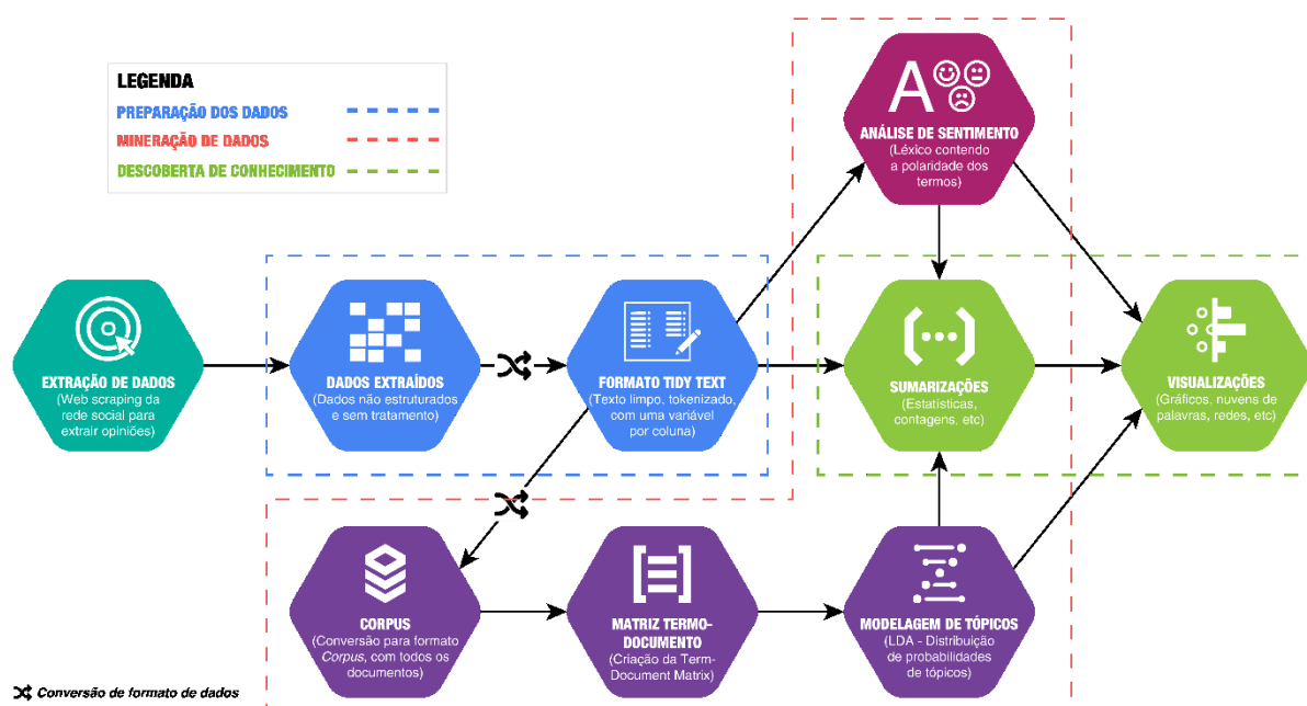
Figura 6 – Framework de Mineração de Opiniões de clientes
