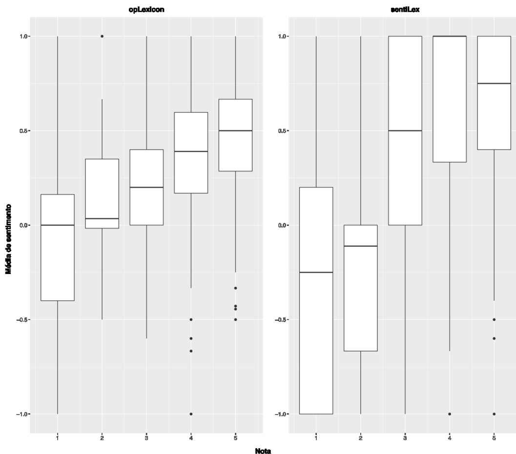
Figura 57 – Média de sentimento por avaliação segundo os léxicos para a EMPRESA 3
