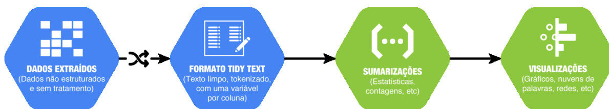
Figura 17 – Esquema da Mineração de Textos aplicado nesta pesquisa
